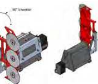
Rechtsanbau am Schlepper
