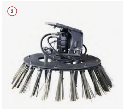
Kunststoffummantelte Stahlseilzöpfe für beste Wildkrautentfernung
