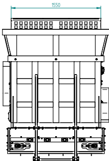
Verarbeitung von ganzen Ballen
